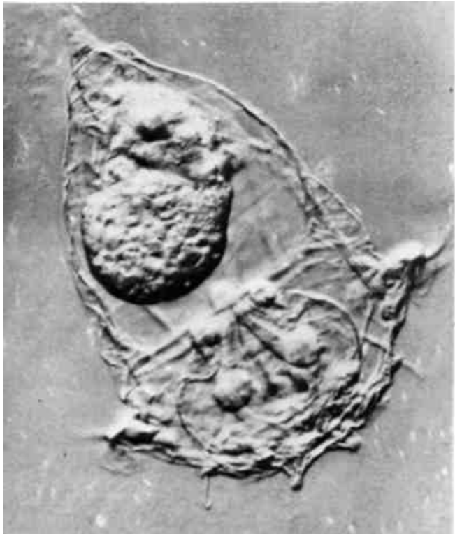
Synchaeta, forma de vida que se alimenta de bactérias; tamanho natural ampliado em 100 vezes.
