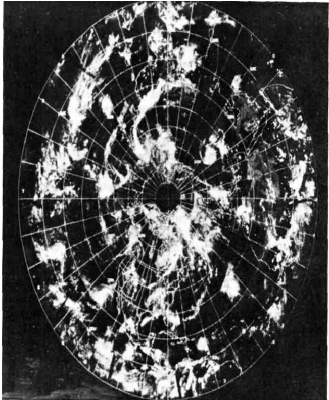
Esta vista compõe-se de um grande número de imagens individuais, tomadas e transmitidas pelo satélite meteorológico ESSA V, em 8-9-1967; sua montagem foi feita mediante um programa de computador. São discerníveis mais de uma dúzia de centros de tempestade e ainda os dos
